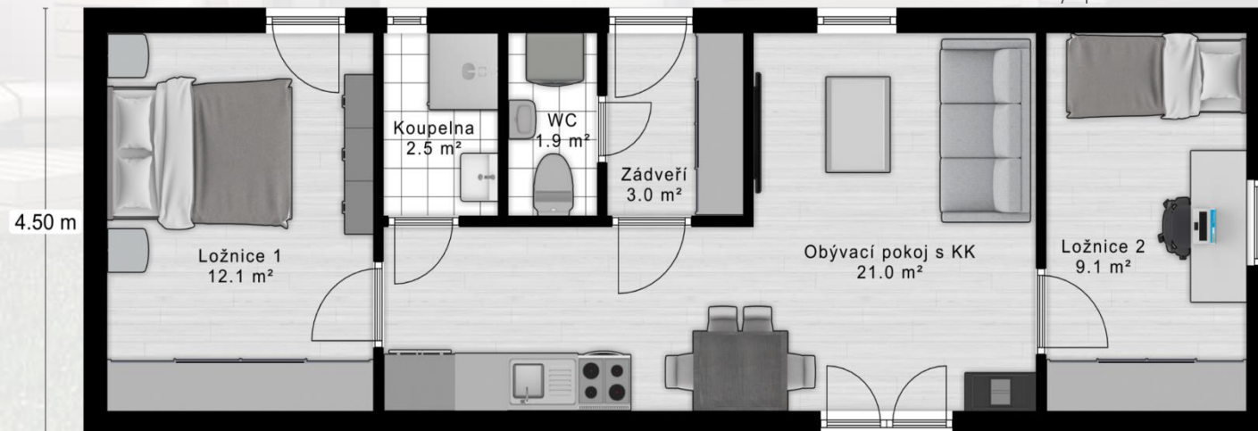
Půdorys přízemí - varianta 2
