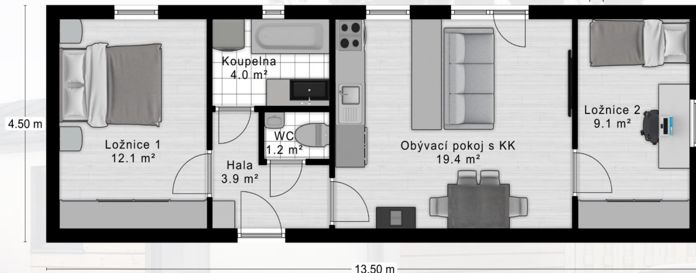
Půdorys přízemí - varianta 2
